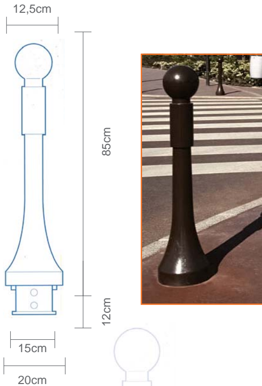
Poller Vega Höhe über Boden 85 cm Gewicht 30 KG
